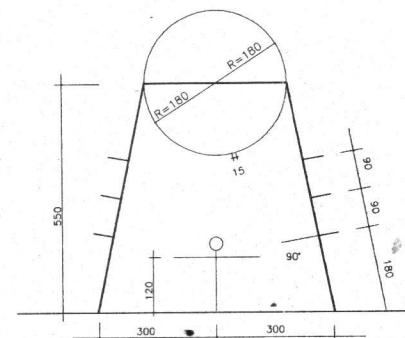
BASQUETEBOL PLANTA-AREA DE LANCE LIVRE ESCALA = MEDIDAS CM
