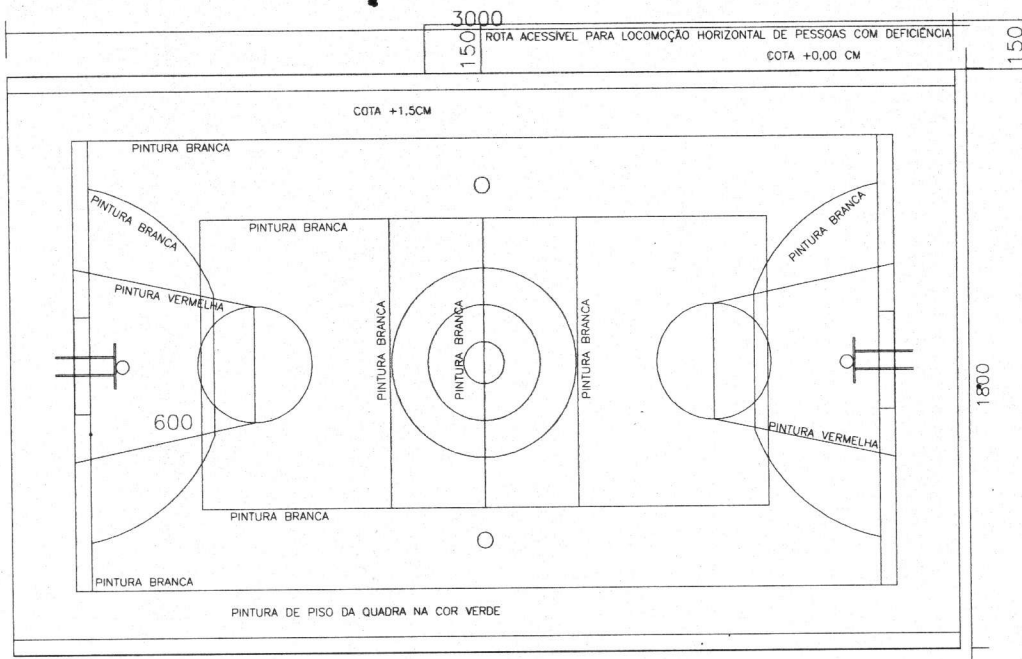
QUADRA POLIESPORTIVA ESCALA=1/100
