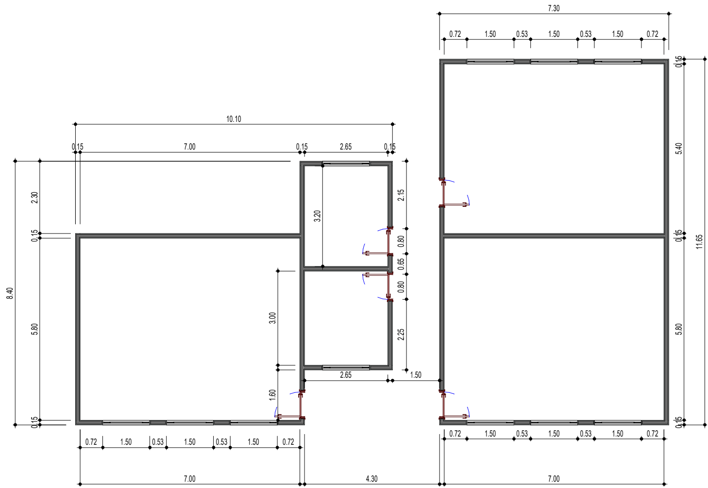
1 PLANTA BAIXA 1 : 100
