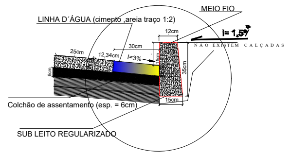
DETALHE 01- MEIO-FIO E SARJETA - BLOQUETE ESCALA 1/10
