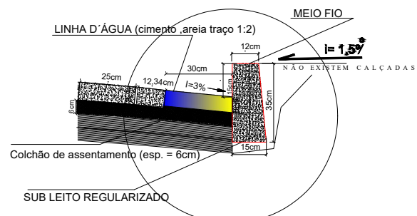
DETALHE 01- MEIO-FIO E SARJETÀ - BLOQUETE ESCALA 1/10
