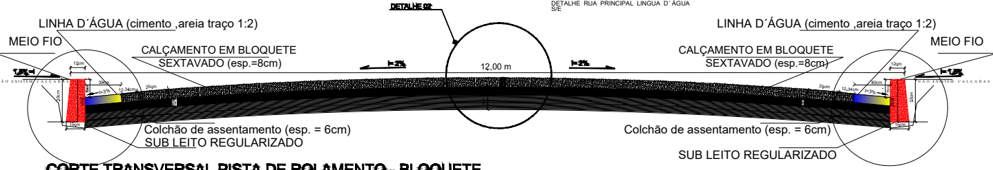
CORTE TRANSVERSAL PISTA DE ROLAMENTO - BLOQUETE ESCALA.....1/20
