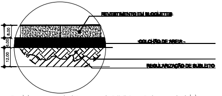
DETALHE 02- CORTE CAMADAS BLOQUETE ESCALA.....1/10
