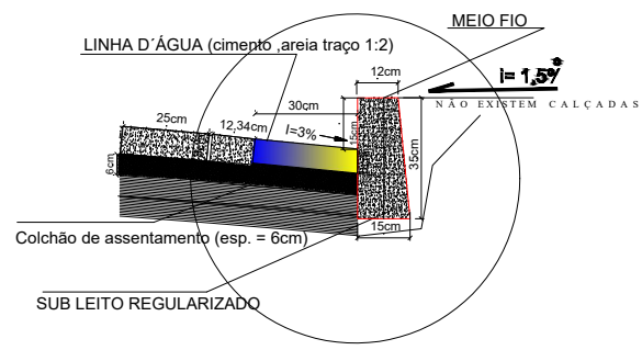
DETALHE 01- MEIO-FIO E SARJETÀ - BLOQUETE ESCALA.....1/10
