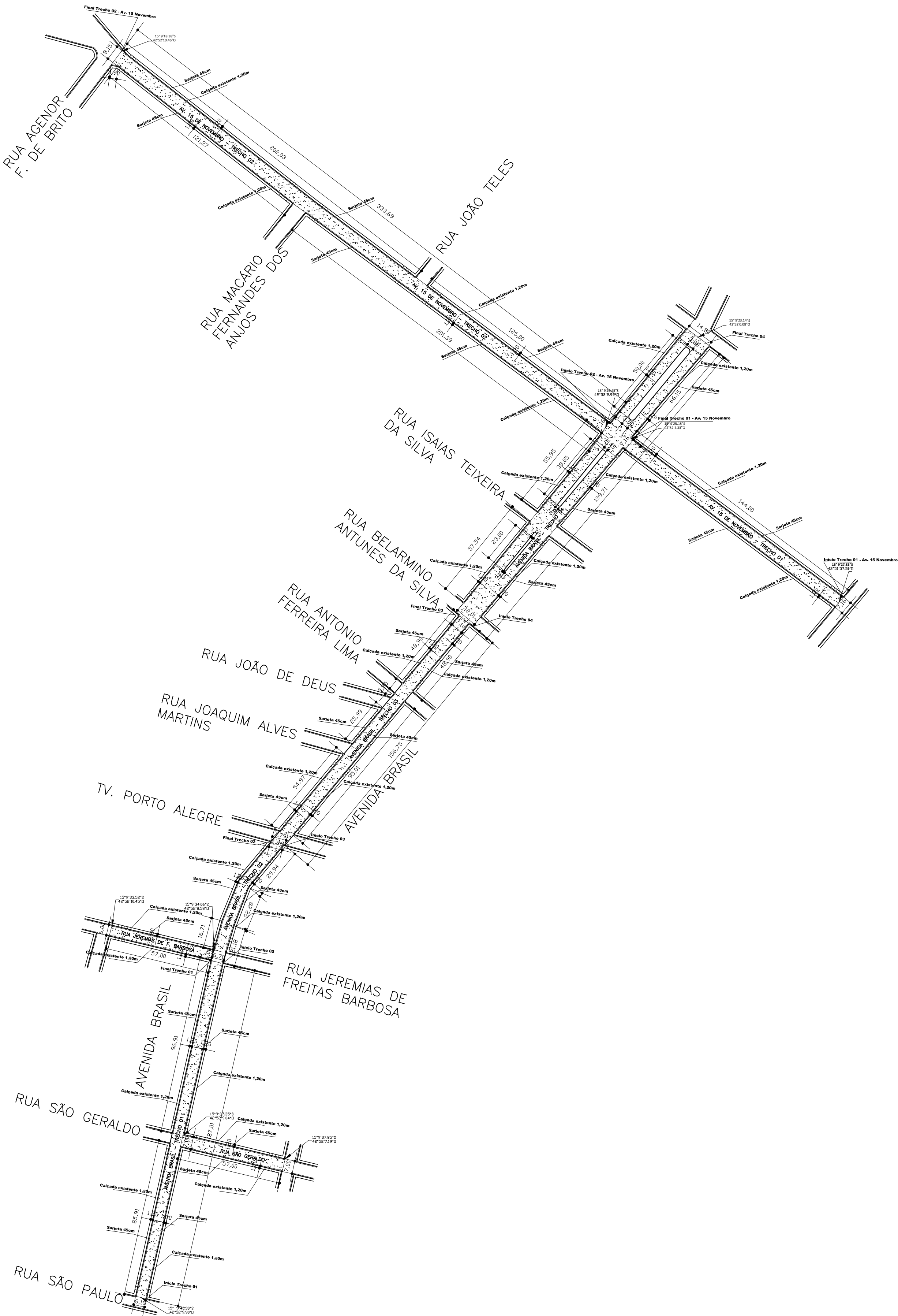
Pavimentação asfáltica Escala.....1/1500
