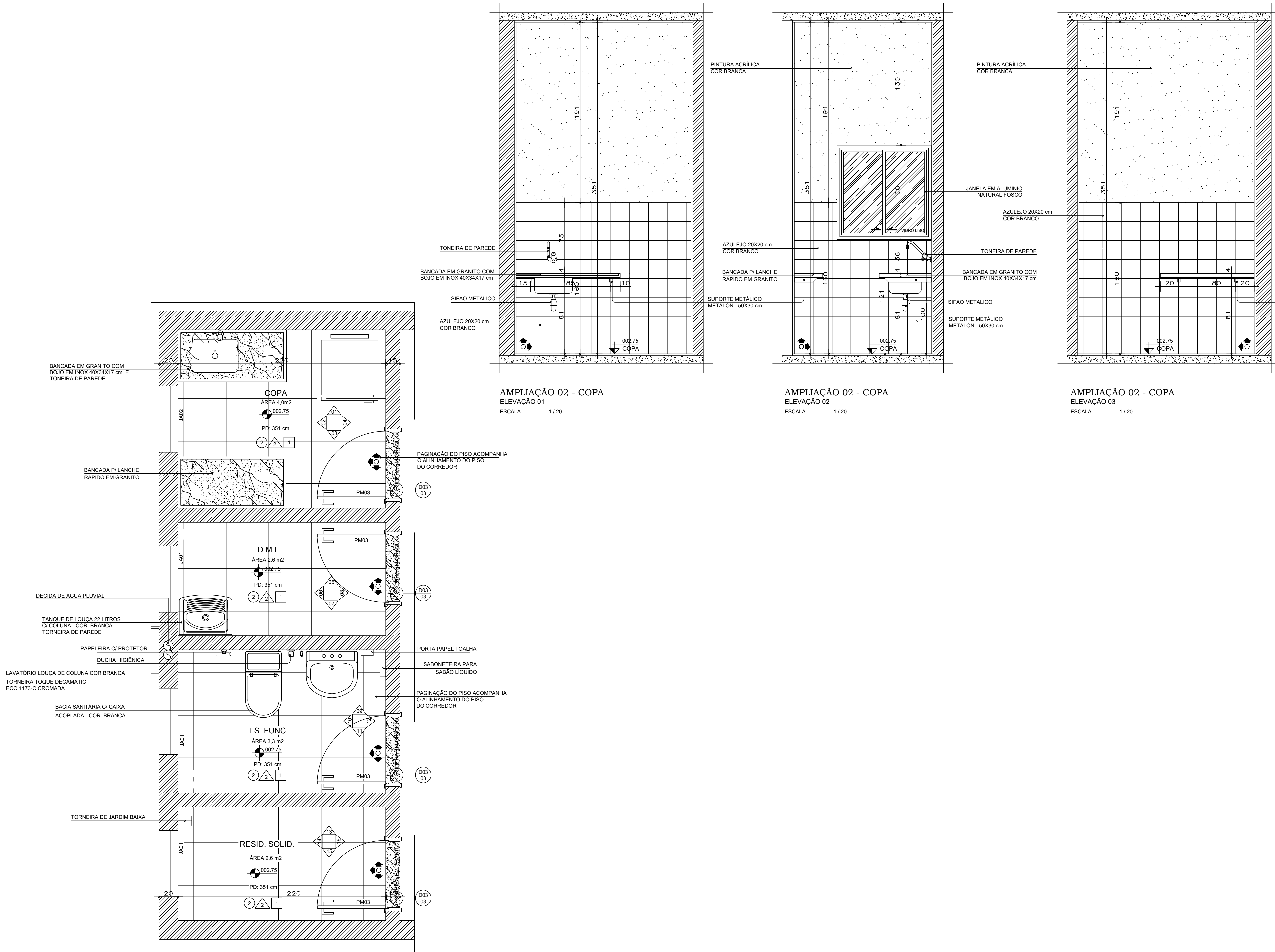
AMPLIAÇÃO 02 - COPA / DML /I.S FUNC./RESID. SOLID. PLANTA ESCALA:.....1 / 20
